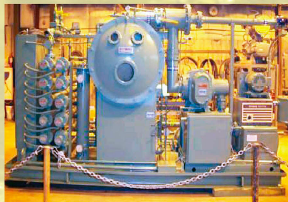
FOTO EJEMPLO DE SISTEMA STOKES 820-20 Y 820-30 DE 20 Y 30 GPM Y SUS BOMBAS
