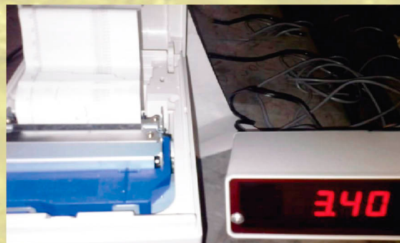
MEDIDOR DIGITAL LUMINOSO, LEE DESDE ATMOSFERA HASTA 1 MICRON VISIBLE DE NOCHE CON IMPRESORA, REGISTRA NUMERICA Y GRAFICAMENTE EL VACIO
